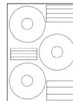
S061160440 rozměr etikety: vnější ø 116 mm vnitřní ø 44 mm Etiket v balení: 300 ks; EAN-kód: 8585026100467
